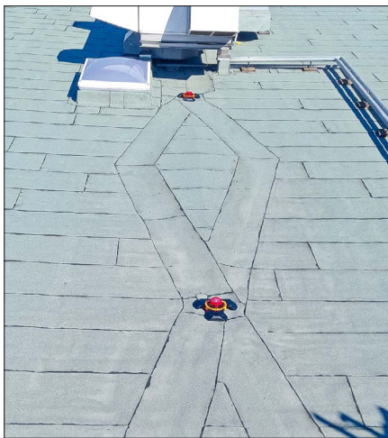
Bild 3: Der Abfluss des Regenwassers erfolgt über Gullys und eine Linienentwässerung in der Mitte der Dachflächen.
